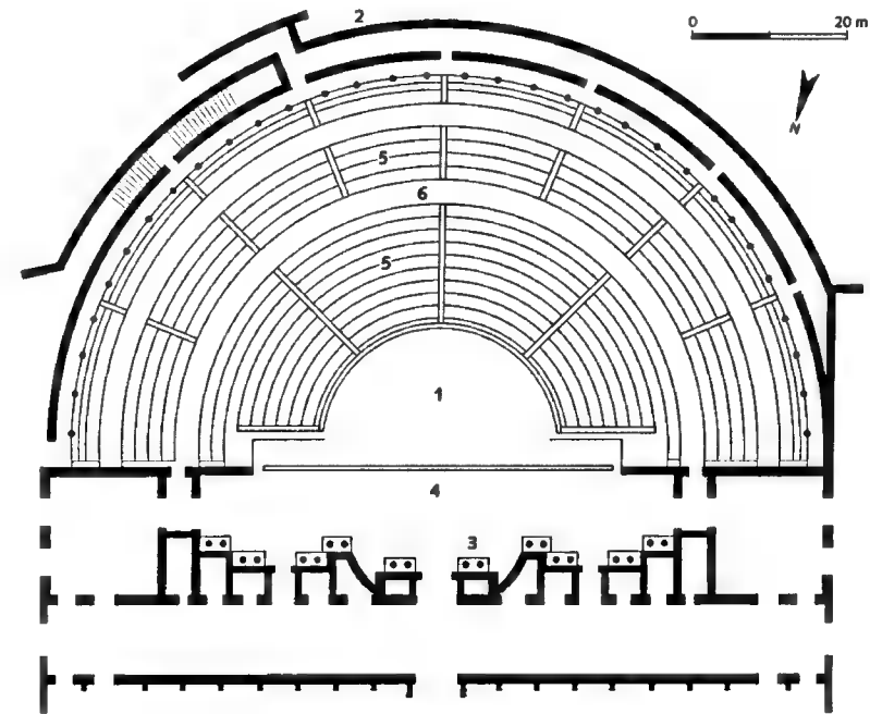
Arausio (Orange), Theater; 1. Jh. n. Chr. (Grundriß). 1 Orchestra/Spielfläche 2 Cavea/Zuschauerraum 3 Scenae frons/Bühnenwand 4 Pulpitum/Bühne 5 Cuneus/Sitzreihenkeil 6 Praeinctio/Gürtelgang
